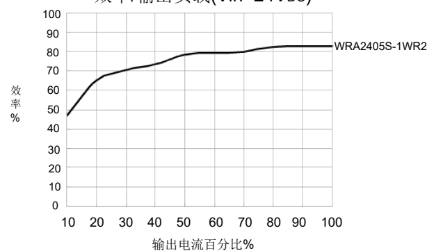
效率/输出负载(Vin=24Vdc)
