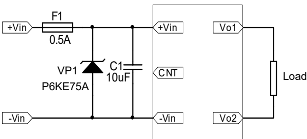
无偏置使用电路
