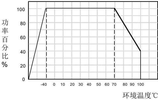
温度/功率降额曲线
