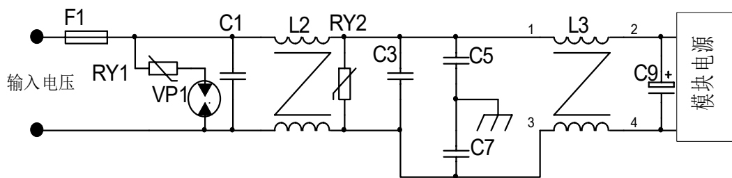
输入滤波和保护电路
