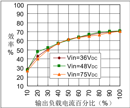
典型效率曲线
